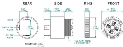
Dimensions
